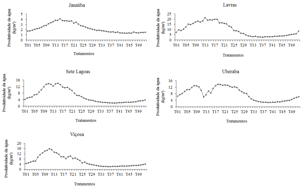
FIGURA 2: Produtividade da água ao longo dos tratamentos para as cinco localidades.
